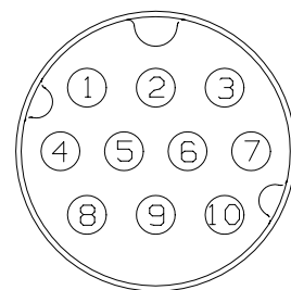
SOLDER LUG VIEW
