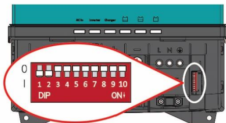
Figure 4 : Commutateurs DIP (réglages usine)
