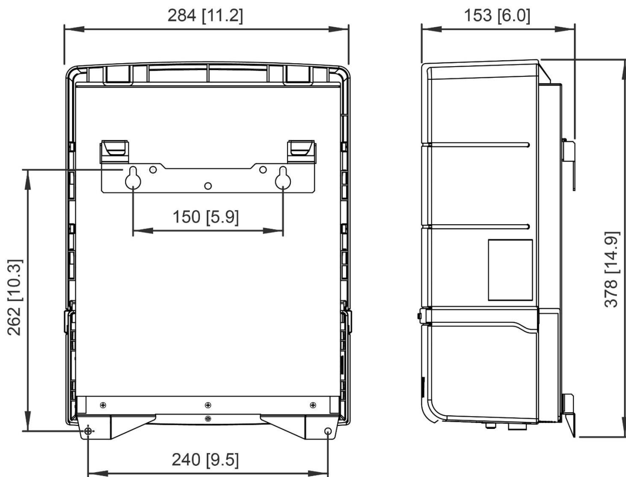
Figure 9 : dimensions en mm [pouces] 12 V/2 000 VA-60 A et 24 V/2 000 VA-40 A
