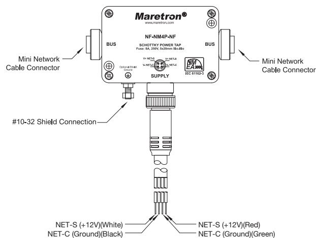
FIGURE 4. Mini Powertap
